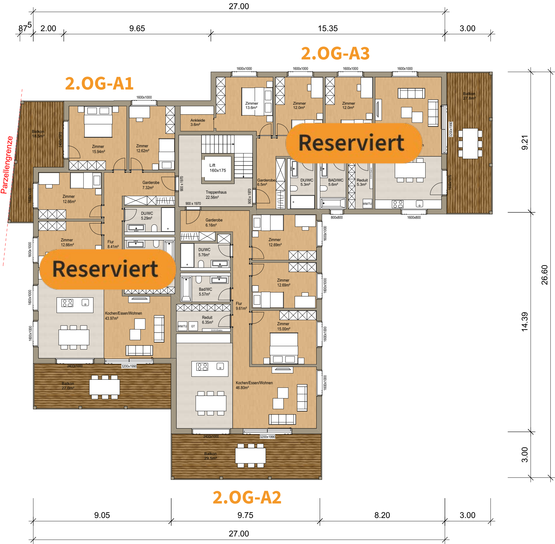
Grundriss 2.Obergeschoss MST:1:150
