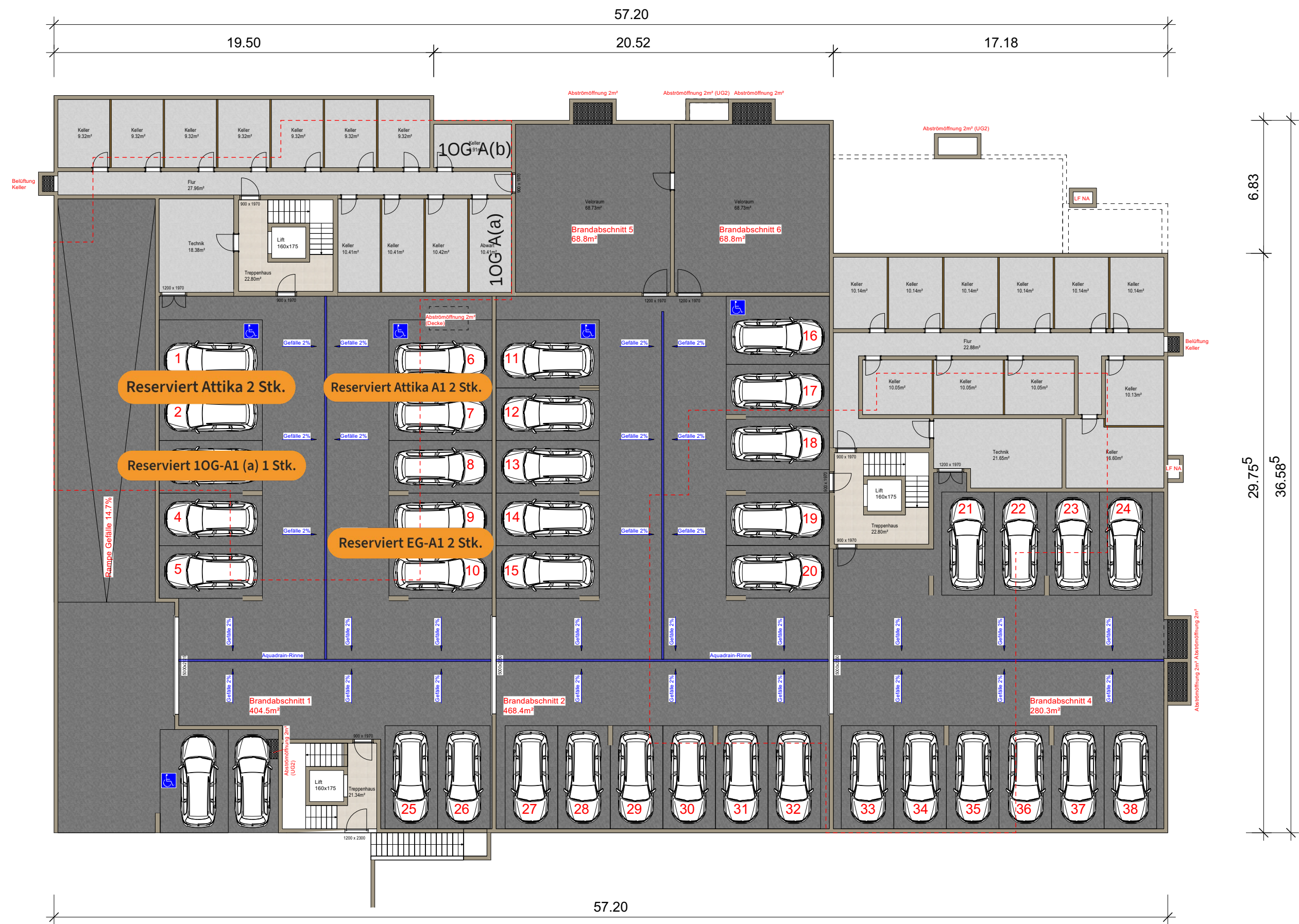
Grundriss 1.UG MST:1:200
