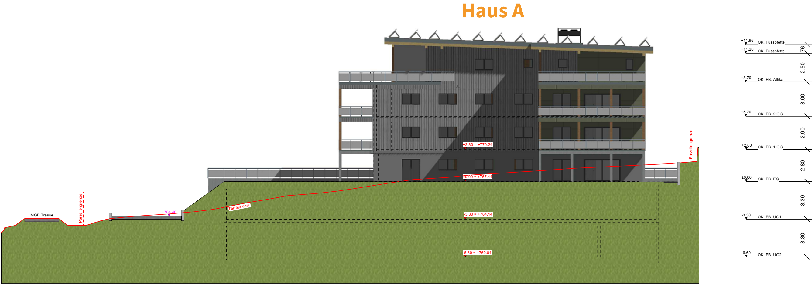
Haus A Fassade Nord-Ost MST:1:200
